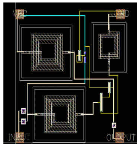
圖 16. 佈局平面圖
